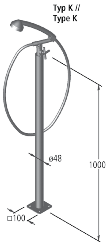
Abb. ohne Entnahmehahn // Drawing without water tap
