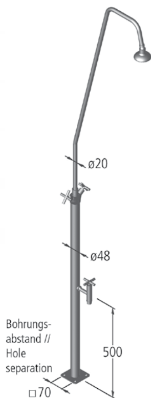
Abb. mit Entnahmehahn // Drawing with water tap
