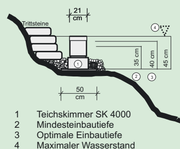
Einbau des Teichskimmers SK 4000 Förderbereich 6 - 12 m³/h
