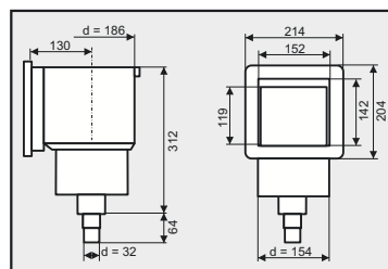
04947 Oberflächenabsauger - Mini - breite Öffnung (20891)
