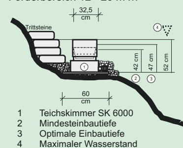
Einbau des Teichskimmers SK 6000 Förderbereich 12 - 20 m³/h
