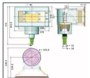
04947 Oberflächenabsauger - Mini - breite Öffnung (20891)
